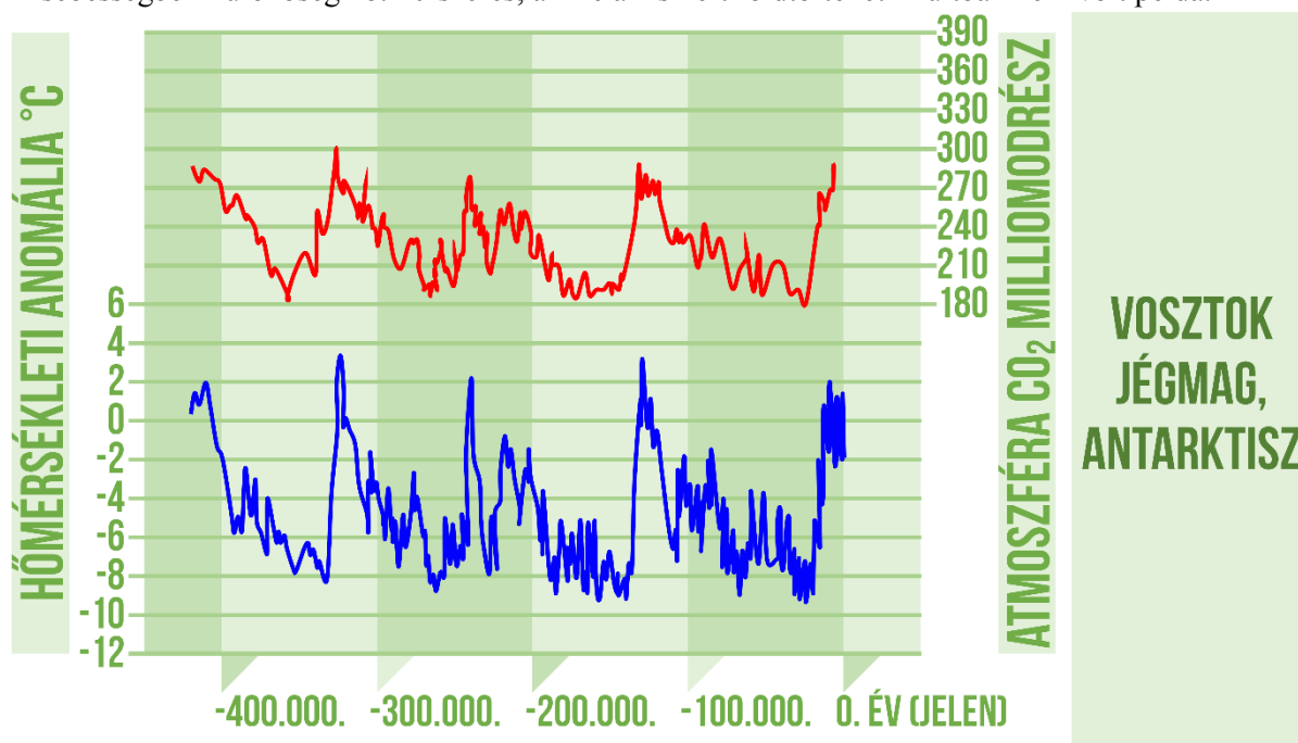
35. ábra: A Vosztok-állomáson vett jégminta (Antarktis) elemzéséből származó hőmérsékleti és CO 2 -adatsor.
